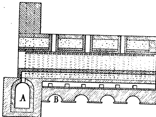
Fig. 23. — Coupe longitudinale.
